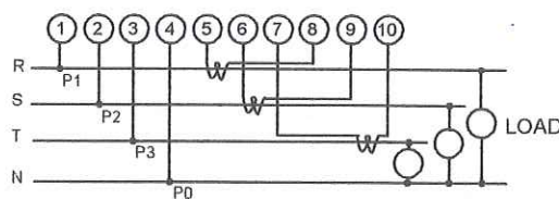
三相四線
