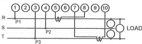
三相三線
