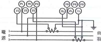
三相二線，併用變比器型
