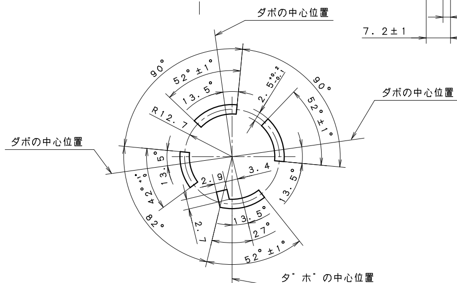
極配置寸法詳細図
