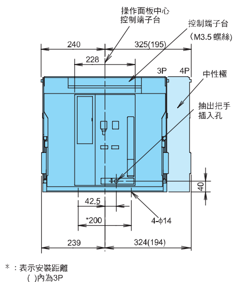
後視圖
