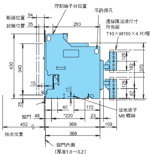
側視圖
