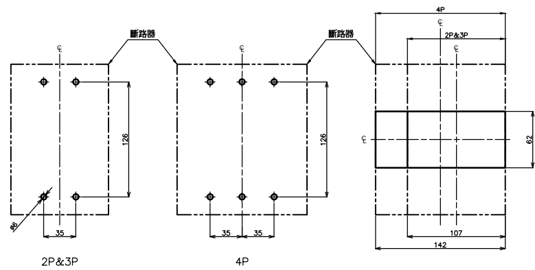
面板尺寸圖
