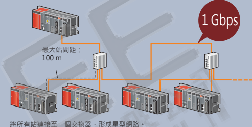
[星型拓撲]
