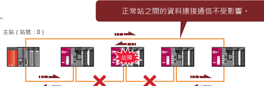
環型拓撲
