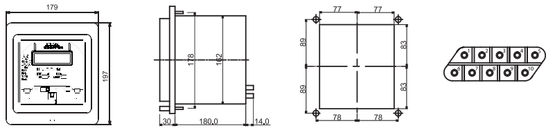
產品尺寸圖/盤面開孔圖/接線端子圖
