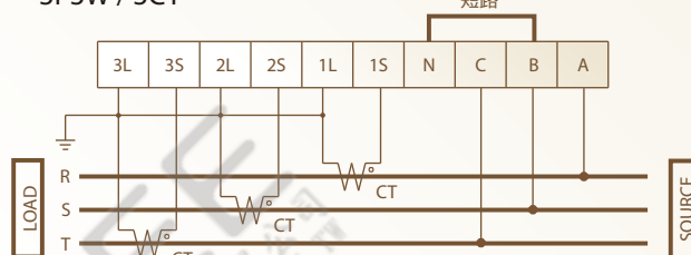
3P3W / 3CT
