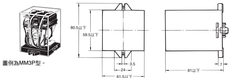
端子配置/內部接線圖 (底視圖)
