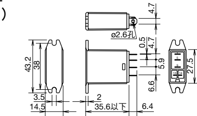
□DPDT 扁平端子型 (頂部凸緣安裝型)
