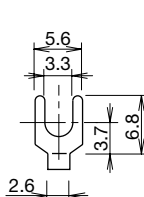
端子部形狀
