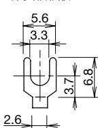
端子部形狀
