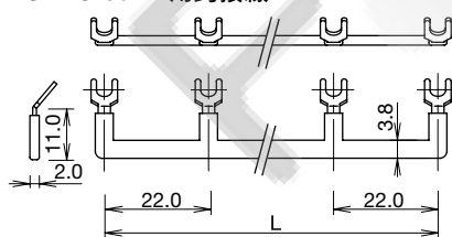
• SM2S-05DF 用跨接線
