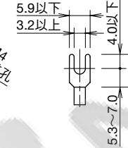
• 適用壓接端子
