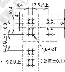
端子配置圖
