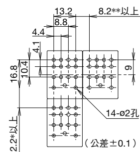
端子配置圖
