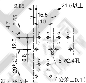
端子配置圖
