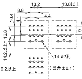
端子配置圖
