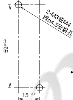
• 安裝孔加工圖
