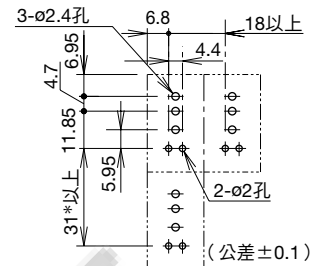
端子配置圖
