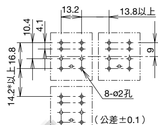
端子配置圖
