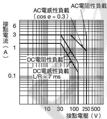
RU4 型（額定負載）
