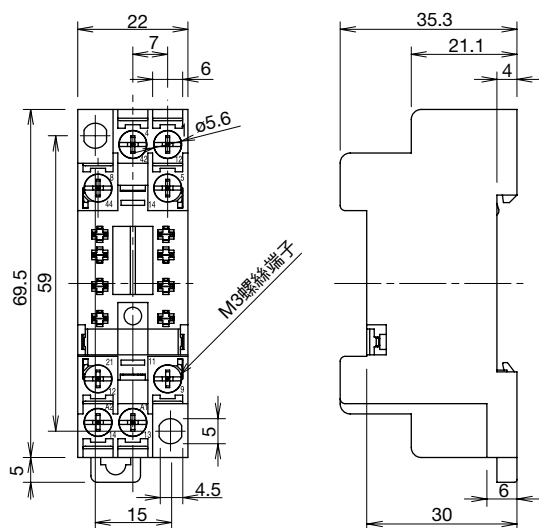
• 端子配置圖
