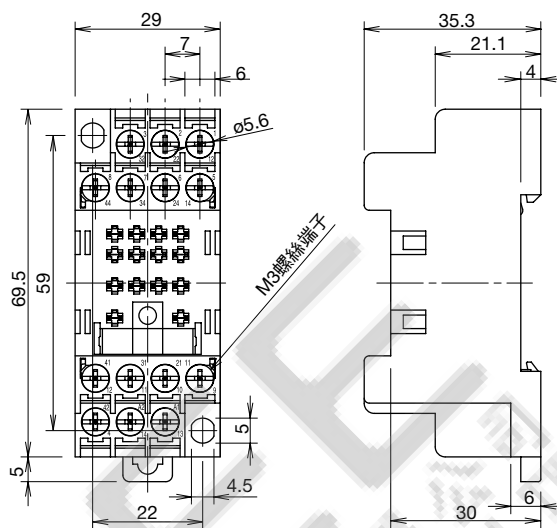
• 端子配置圖
