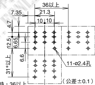
端子配置圖
