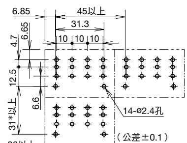
端子配置圖
