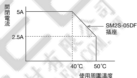
降低額定值遞減特性圖
