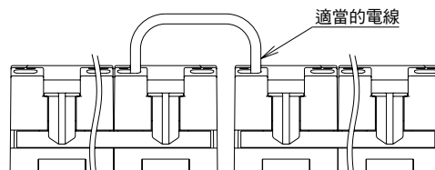
相鄰插座間 #14 端子的跨接線的接線
