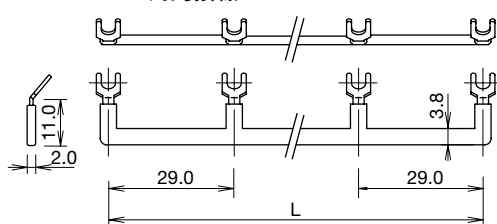
• SY4S-05DF 用跨接線
