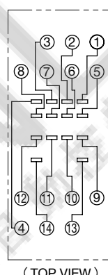
• 端子配置圖
