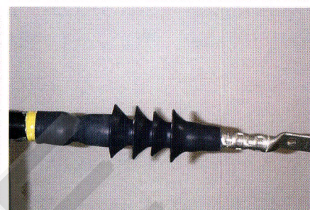
3. 拉完支撐管後，安裝完成
