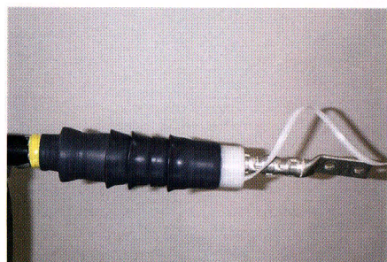
2. 將QT-III定位後拉掉白色支撐管
