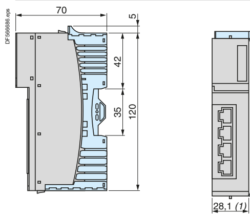
Parallel wiring module Advantys STBEPI2145
