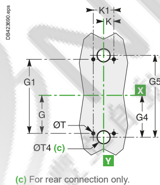
1 pole
