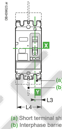
2 poles
