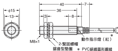
圖3 E2E-X1R5Y□型
