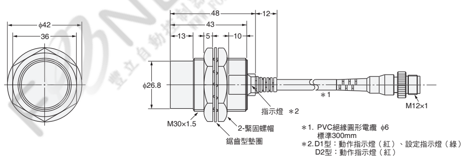
圖33 E2E-X20MD1-M1GJ型 E2E-X20MD1-M1TGJ型 E2E-X20MD□-M1TGJ-US型
