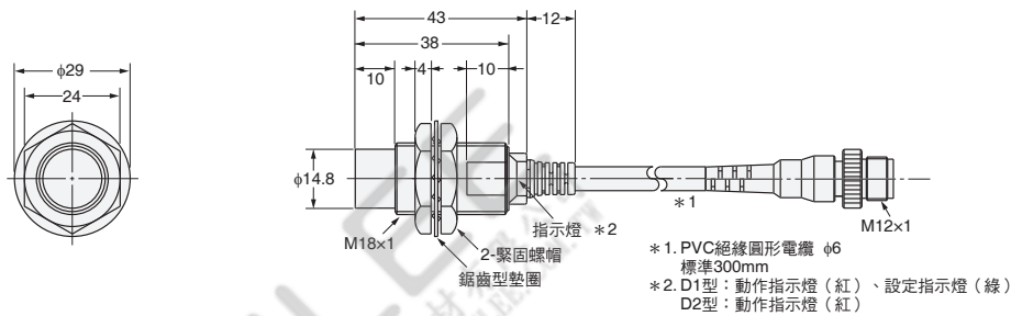
圖32 E2E-X14MD□-M1GJ型 E2E-X14MD1-M1TGJ型 E2E-X14MD□-M1TGJ-US型
