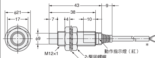
圖8 E2E-X5MY□型
