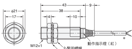
圖7 E2E-X2Y□型
