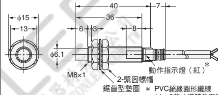
圖4 E2E-X2MY□型
