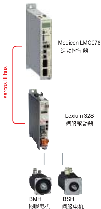
采用 Sercos III 运动控制总线的控制系统架构示例
