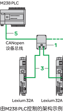
由M238 PLC控制的架构示例
