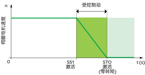
“安全停止1” (SS1) 安全功能的激活
