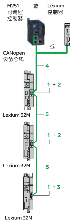
通过 VW3 A3 618 卡将伺服连接到 CANopen 网络示例
