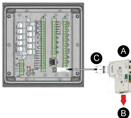
Figure 193 - VSE-001 module
