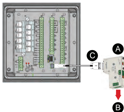
Figure 194 - VSE-002 module
