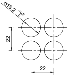
圆形 (LB6P/LB6MP 型)
