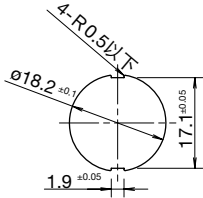
可决定位置的面板切割尺寸 圆形 (LB6P/LB6MP 型)
