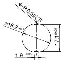
□可决定位置的面板切割尺寸 圆形 (LB6B/LB6MB/LB6GB 型)
