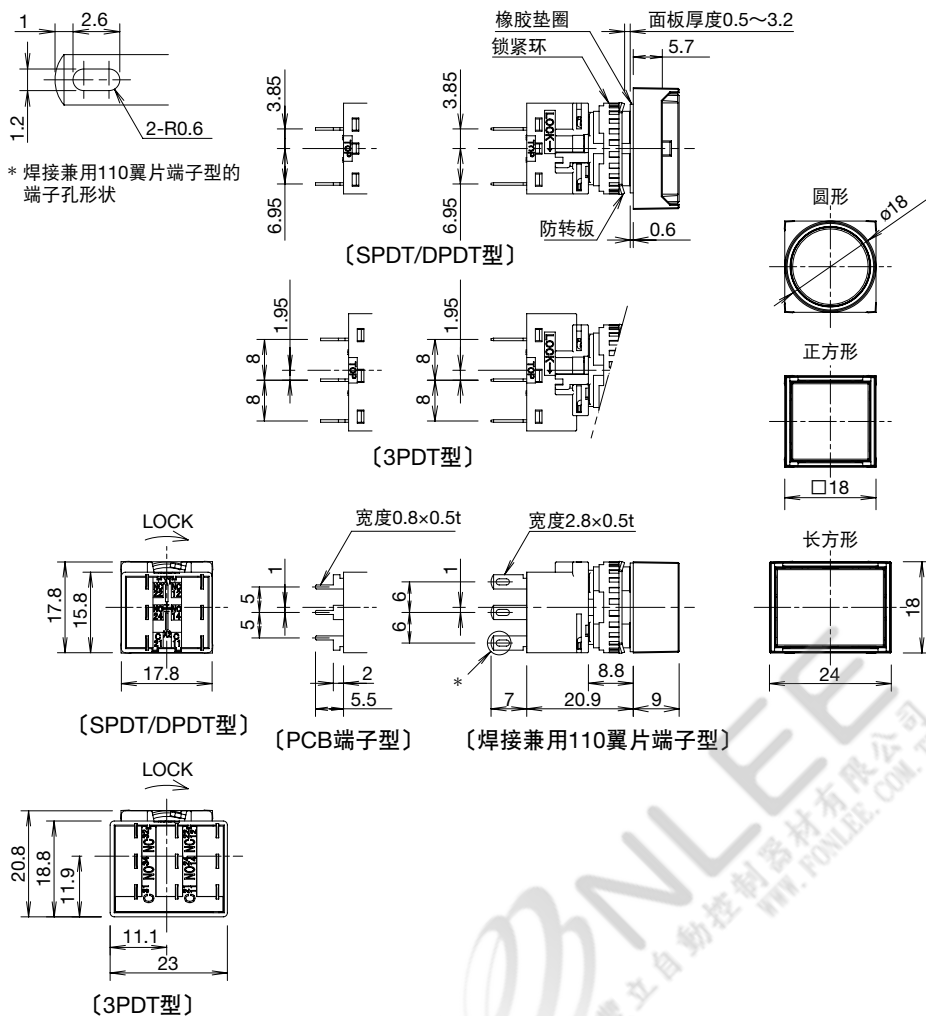
SPDT/DPDT 型 TOP
