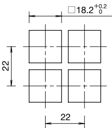
正方形 (LB7P/LB7MP 型)
