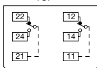
SPDT/DPDT 型 TOP
