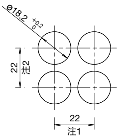
□安装孔加工图·最小安装中心间距
