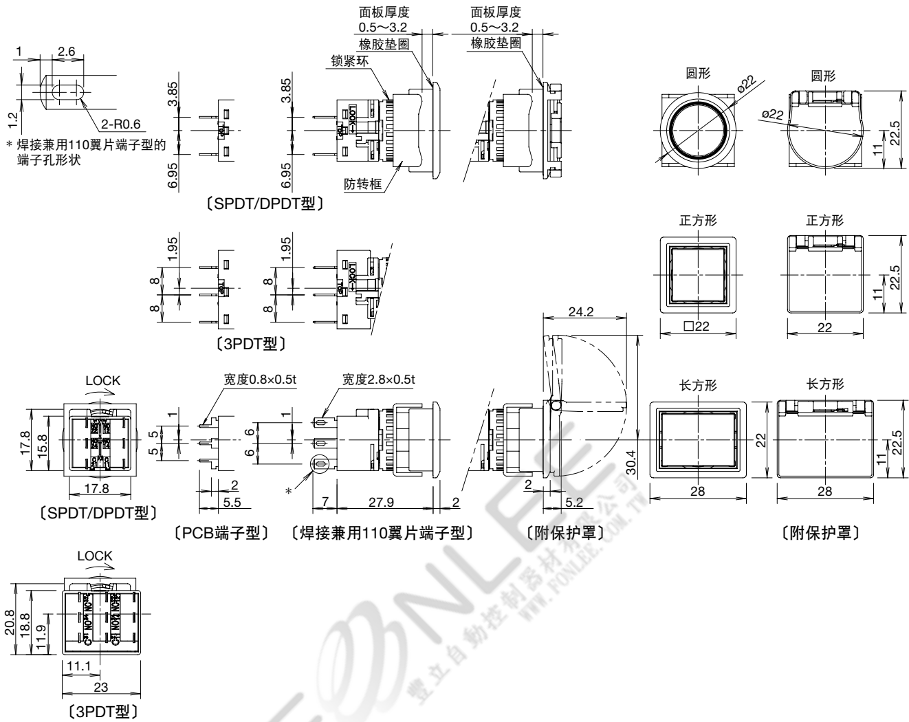
□端子排列图 (BOTTOM VIEW) SPDT/DPDT 型 3PDT 型
