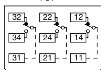
3PDT 型 TOP
