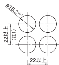
LB7/LB7M/LB7G 型
