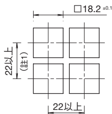
LB7/LB7M/LB7G 型
