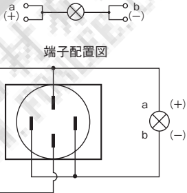
回路図
