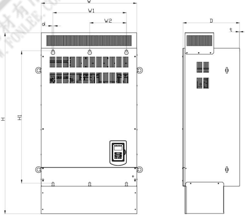
外型圖 G
