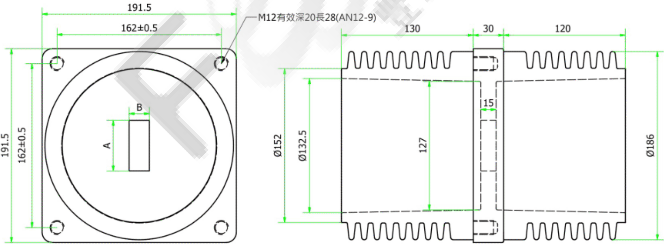
開口尺寸表
