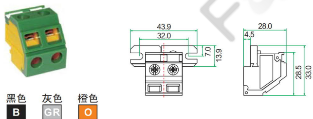
MTB 系列端子台參數一覽表
