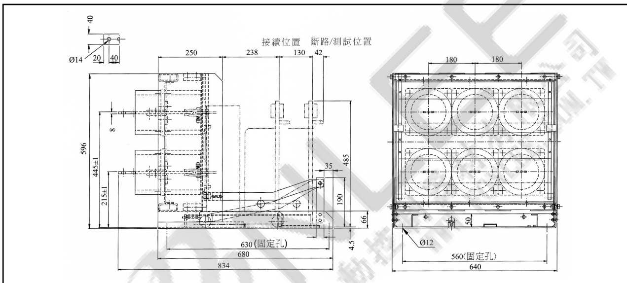
■ 斷路器外觀尺寸圖 套管式抽出型
