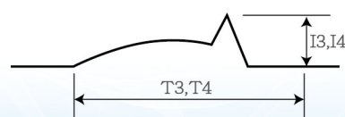
(註二) 閉路，開路控制電流時間特性
