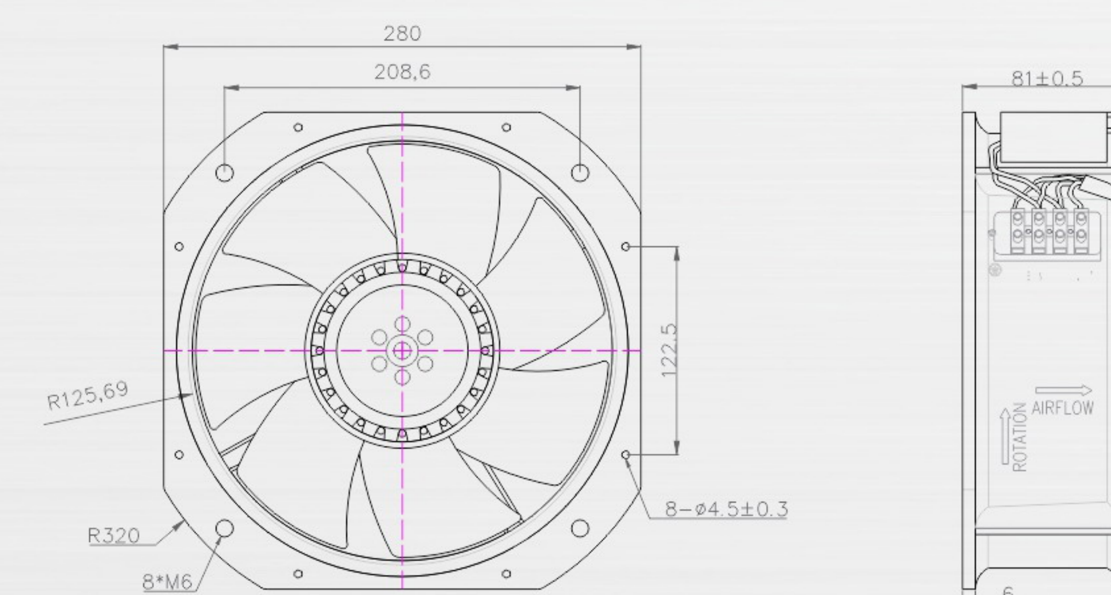
> External Dimension(mm) 外型尺寸(mm)
