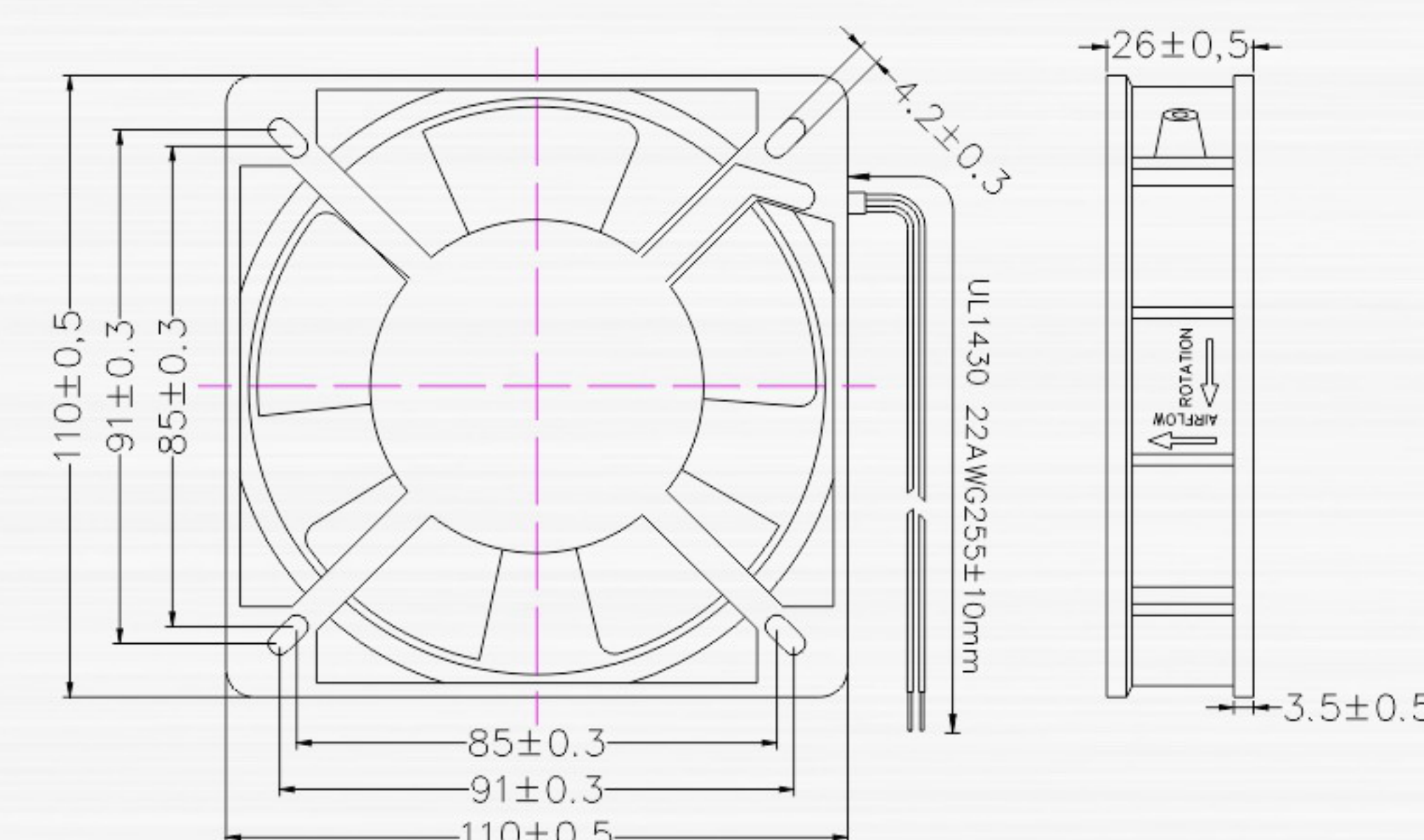
> External Dimension(mm) 外型尺寸(mm)
