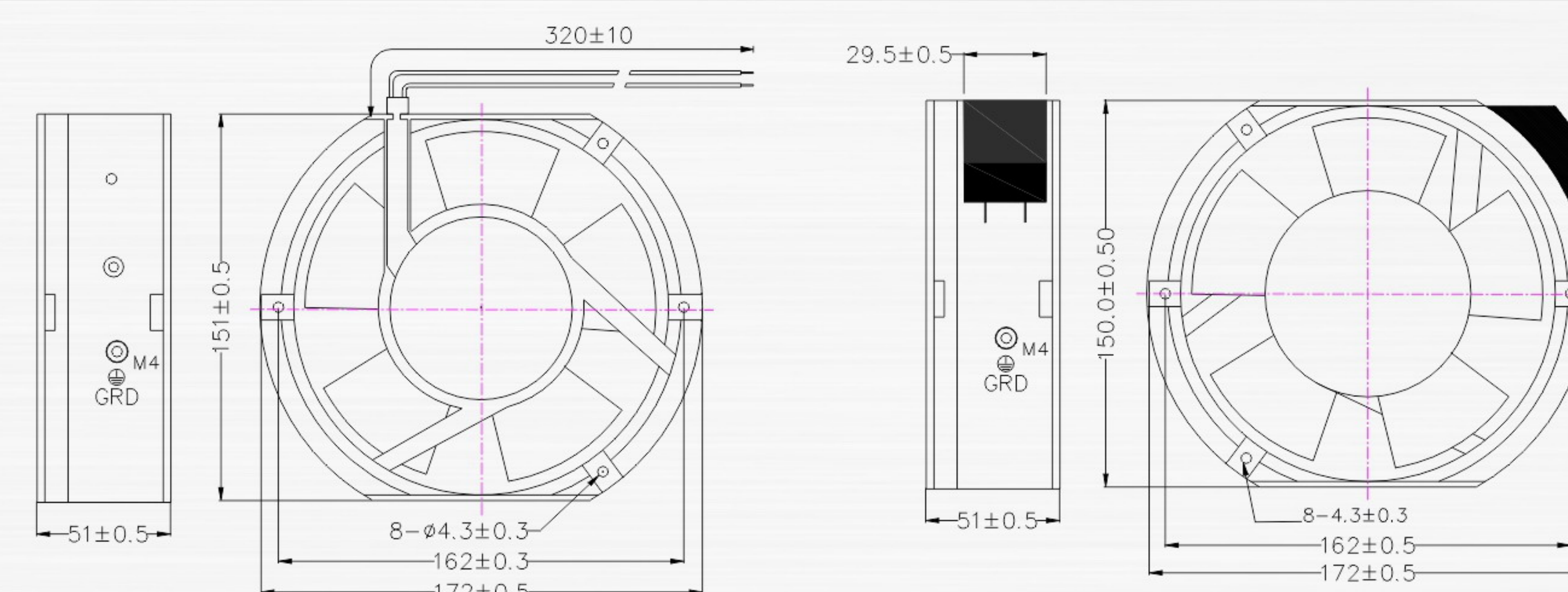
> External Dimension(mm) 外型尺寸(mm)
