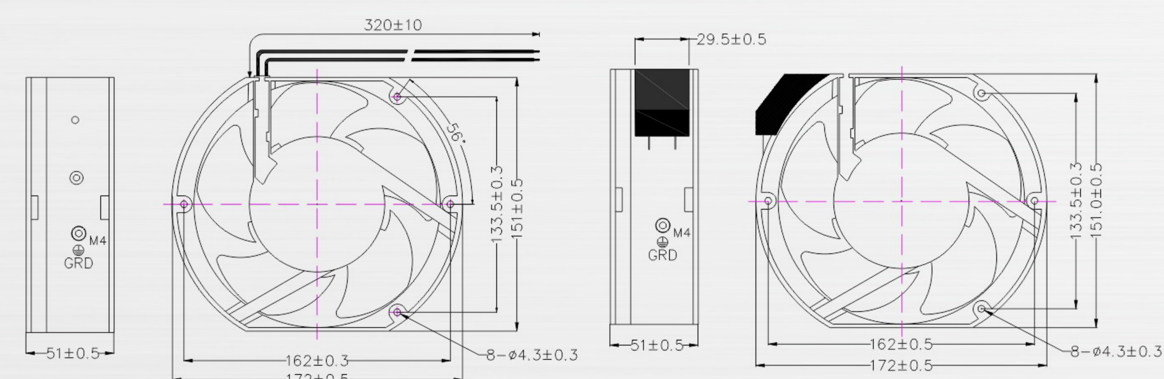
> External Dimension(mm) 外型尺寸(mm)
