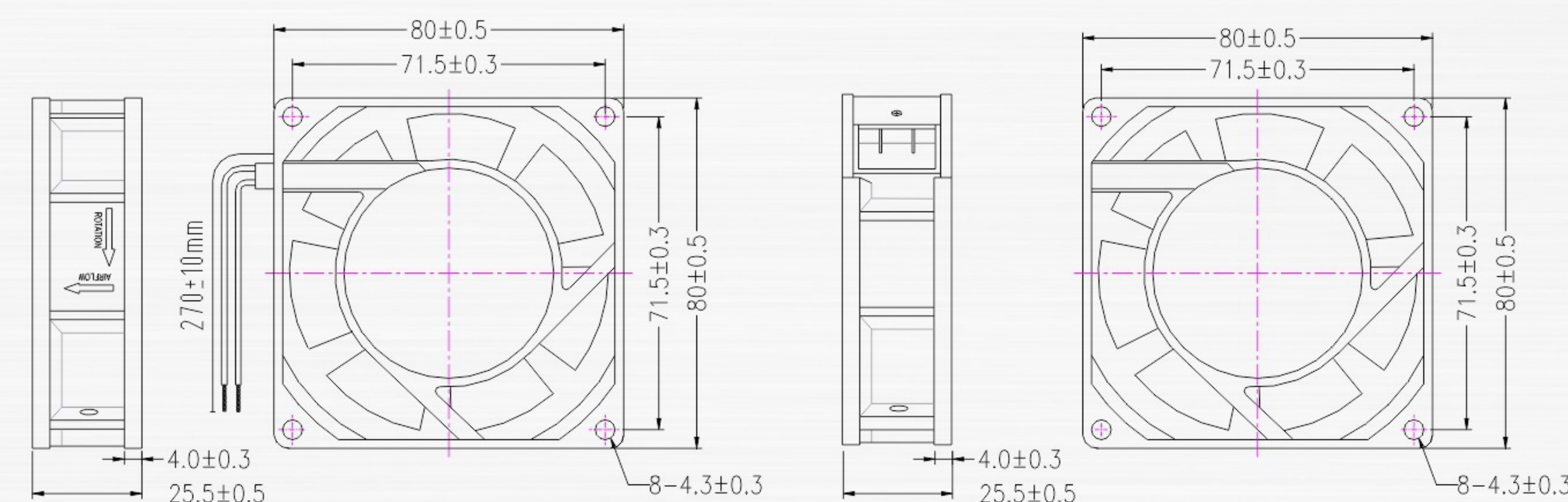
> External Dimension(mm) 外型尺寸(mm)
