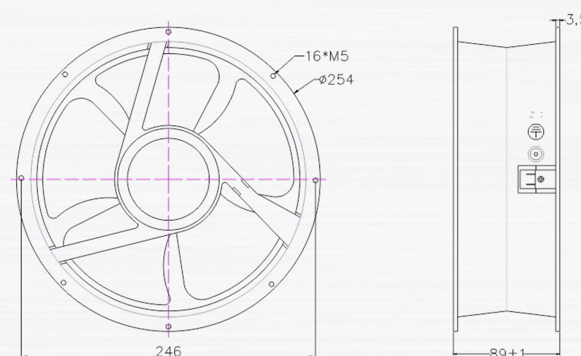
> External Dimension(mm) 外型尺寸(mm)
