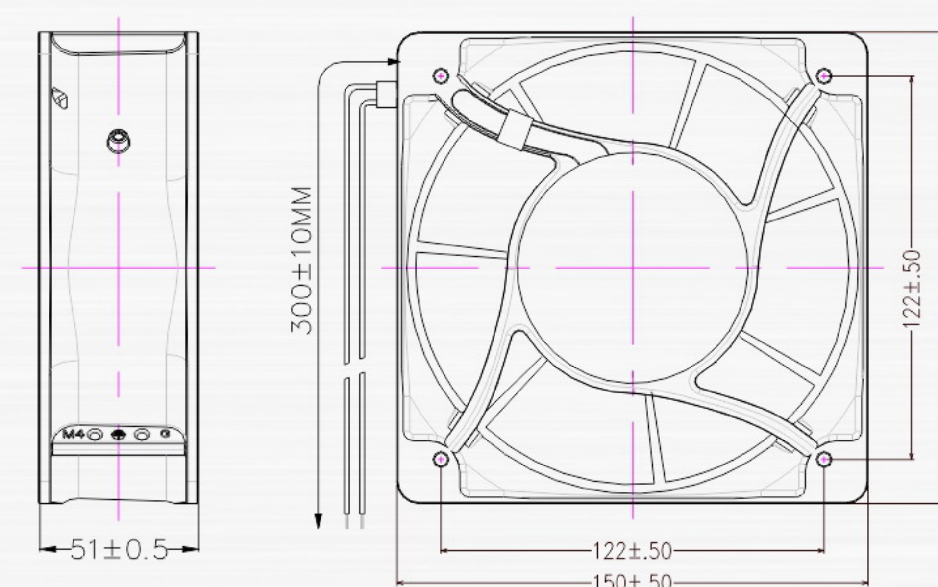
> External Dimension(mm) 外型尺寸(mm)
