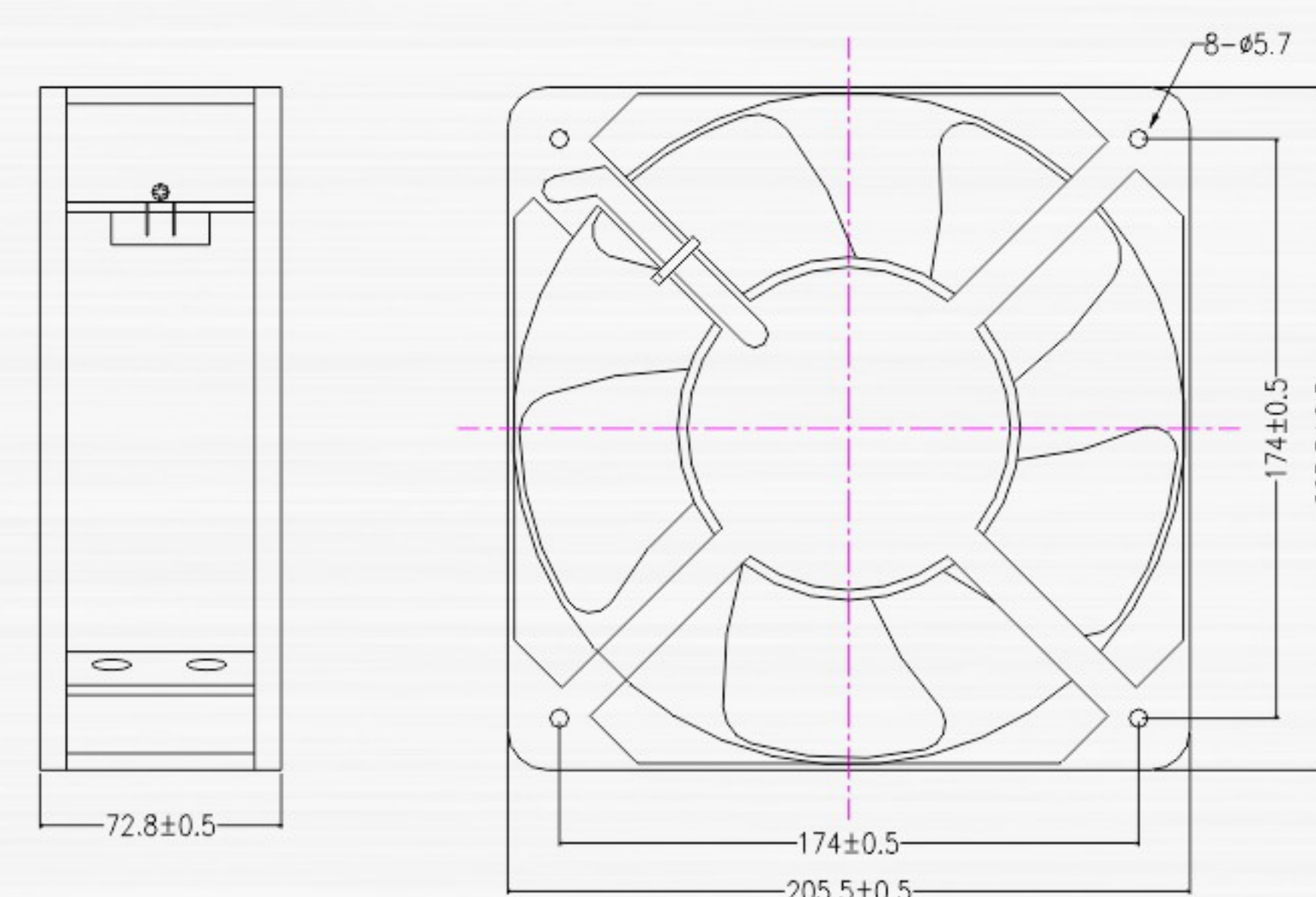
> External Dimension(mm) 外型尺寸(mm)
