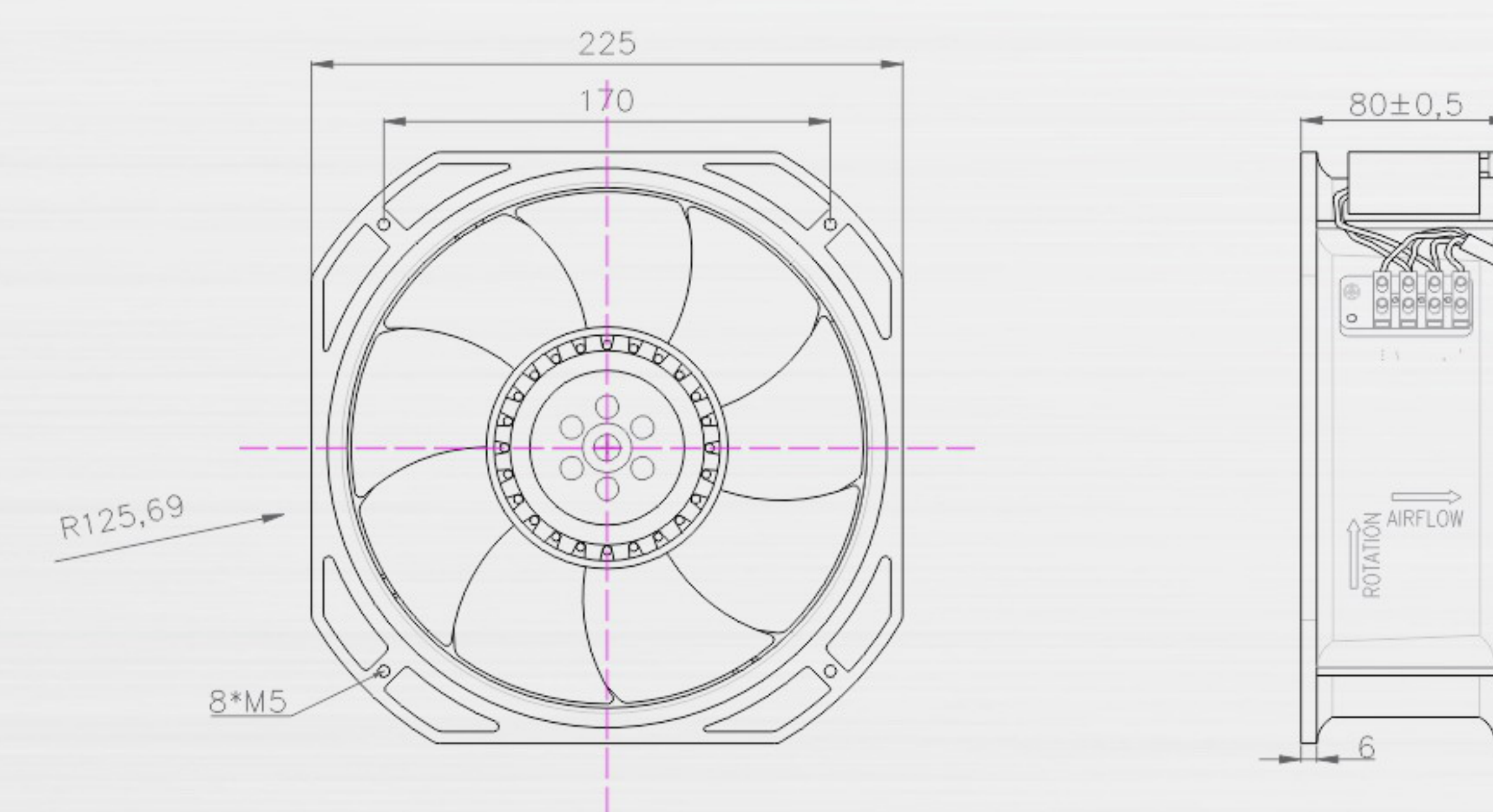
> External Dimension(mm) 外型尺寸(mm)
