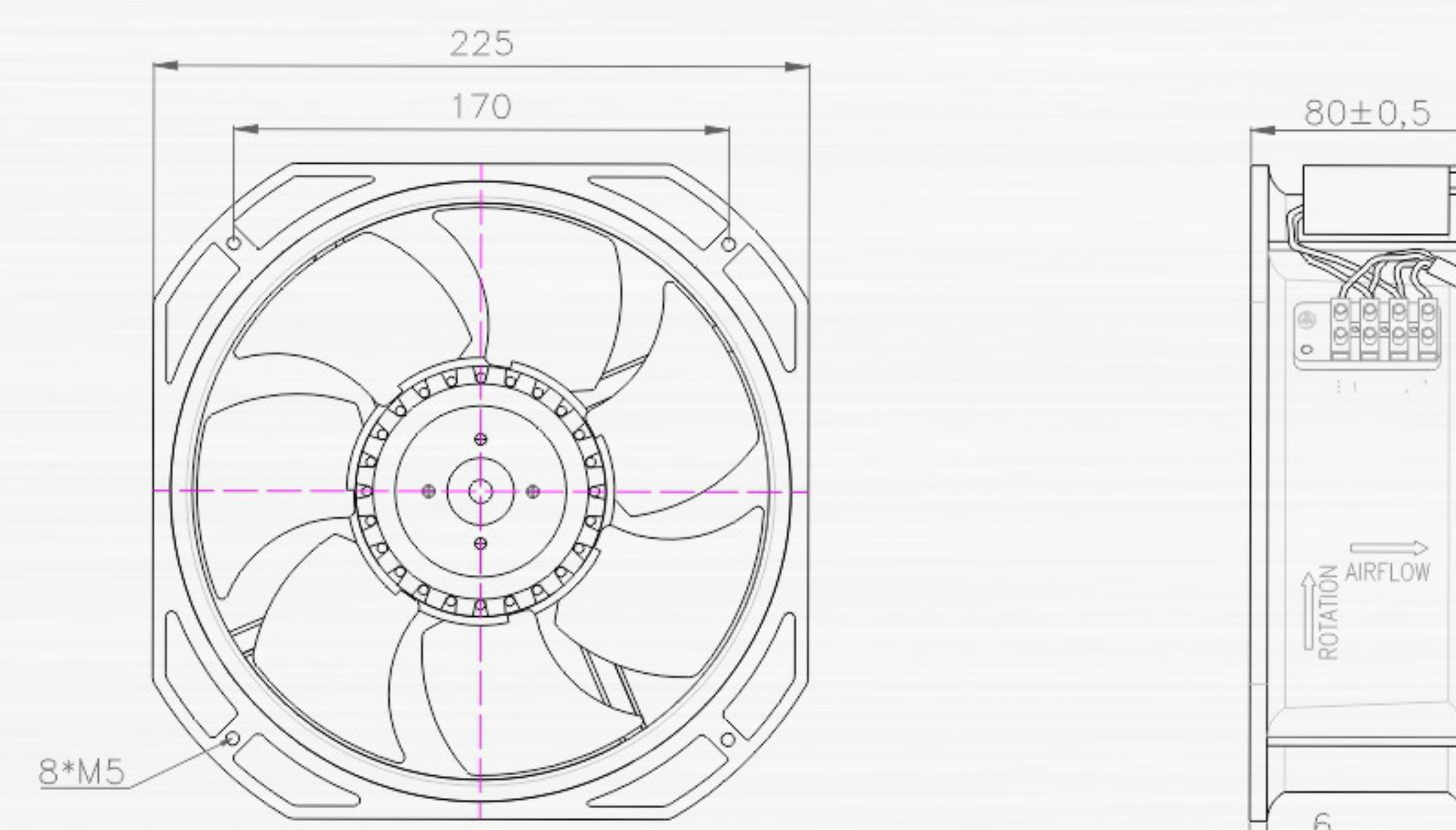
> External Dimension(mm) 外型尺寸(mm)
