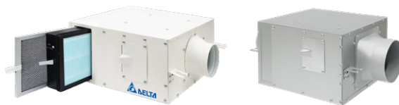
全室淨化新風機 / 負壓排氣型管道扇 安裝便利、輕鬆省事
