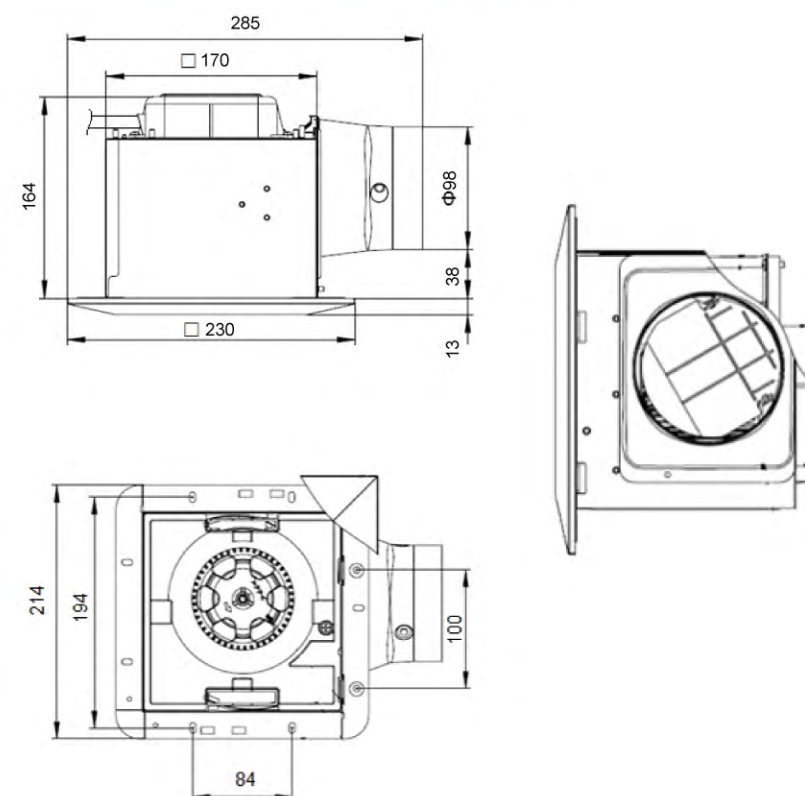
FV-17CU8R / FV-17CU8W 設計·施工用圖
