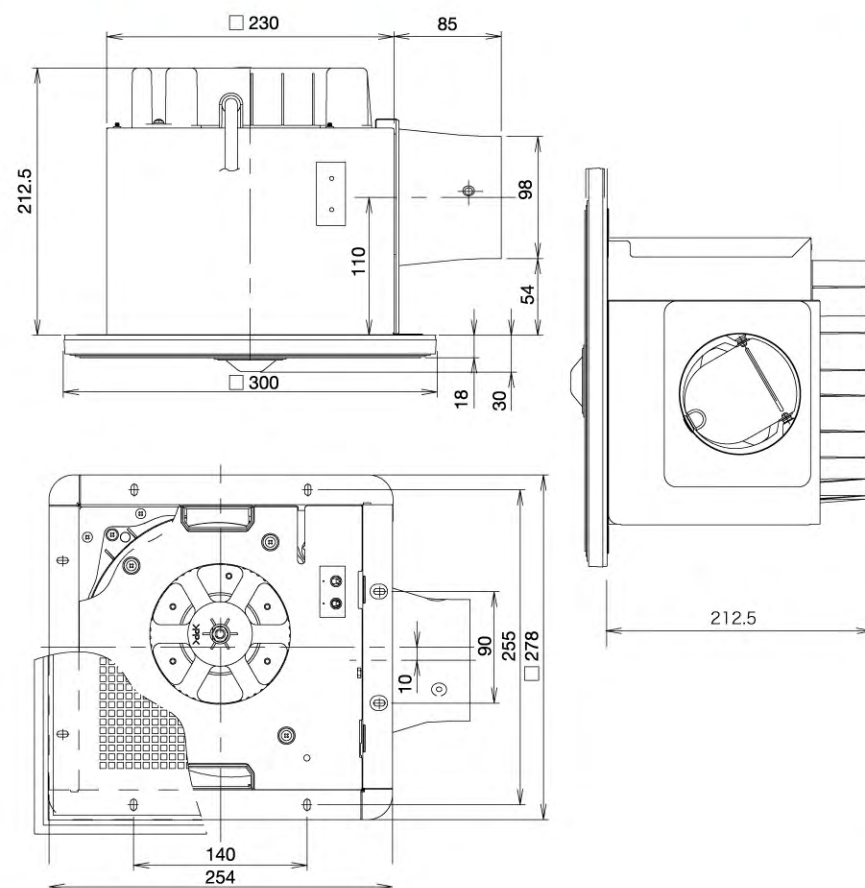
FV-24JA2W 設計·施工用圖
