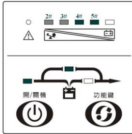
↑ 圖3-7 輸入接電源線限制容量設定
