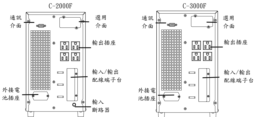
↑ 圖 1-2 C-2000F、C-3000F 後蓋板
