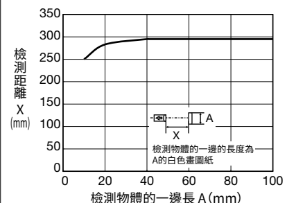
●檢測距離—檢測物體大小特性
