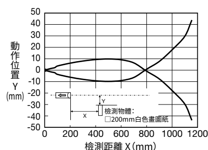
●動作範圍特性
